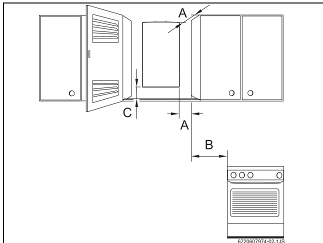
Fig. 7 Distanțe minime
