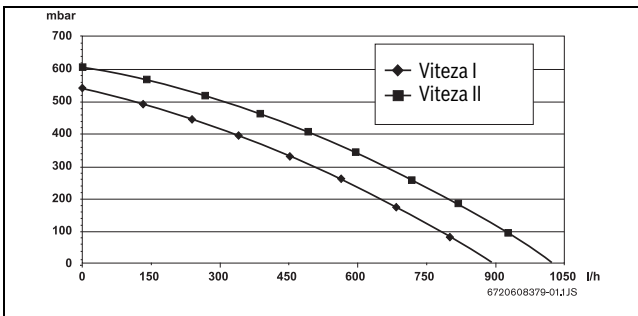
Fig. 6 Caracteristica pompei
