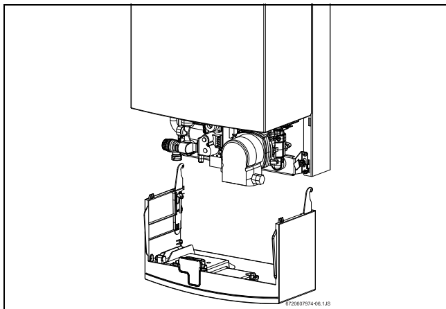
Fig. 11 Scoaterea panoului de comanda
