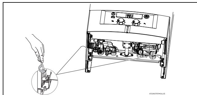
Fig. 9 Șuruburi de siguranță
