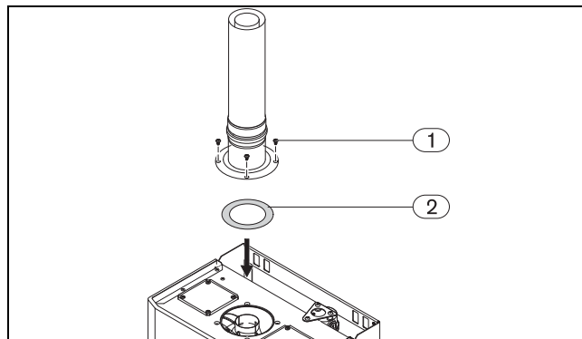
Fig. 14 Montare diafragma de laminare
