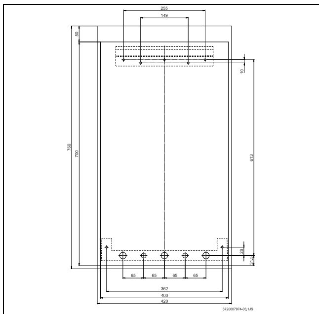
Fig. 8 Ansamblu de montare pe perete
