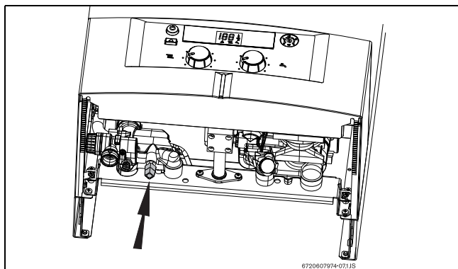
Fig. 16 Robinet de umplere
