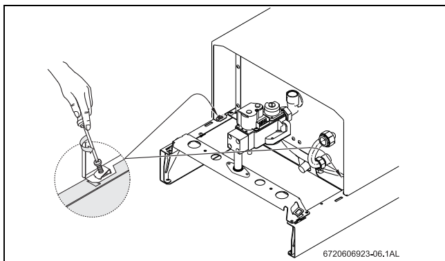
Fig. 12 Se scoate mantaua
