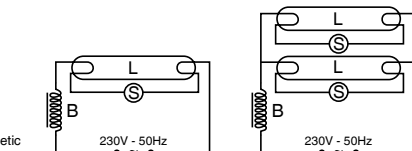
Schita montaj pentru tub fluorescent T8 18W cu balast electromagnetic 1x18W si 2x18W
