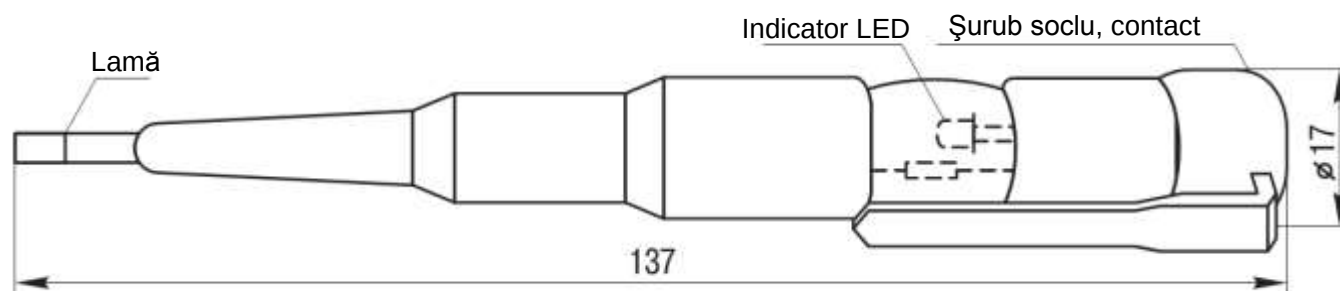
Fig.1 Șurubelnița tester tip OP-1
