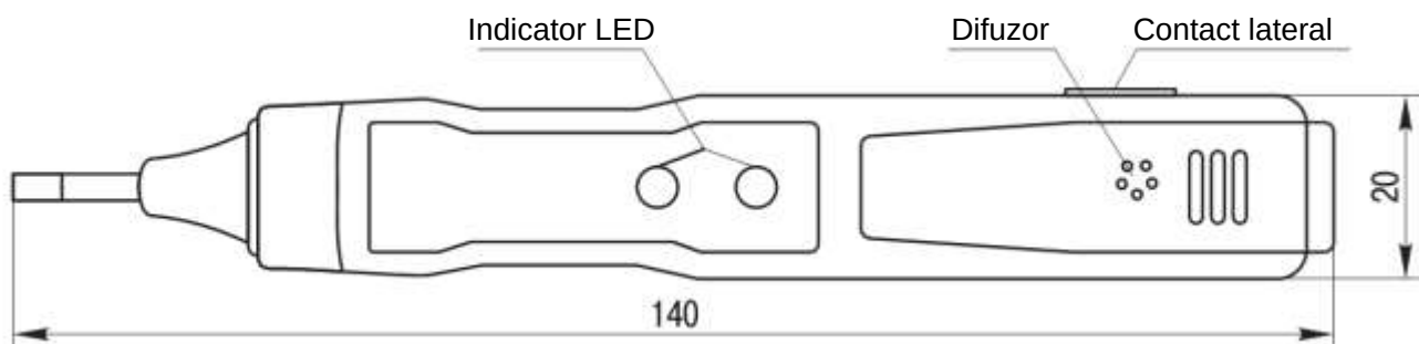
Fig.1 Șurubelnița tester tip OP-1
