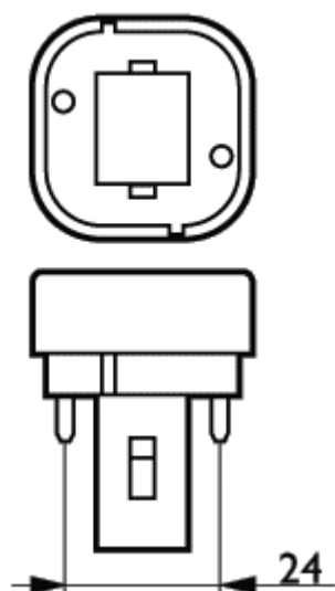
Soclu/Baza G24d-2
