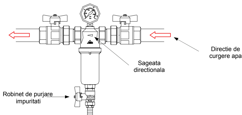
Schema de montaj a filtrului cu curățare prin purjare
