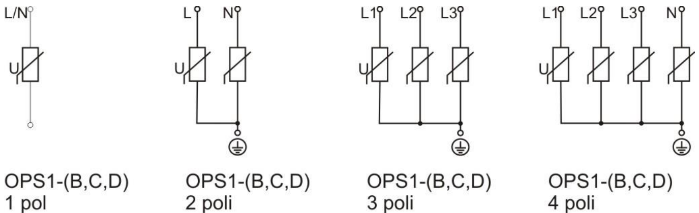
Fig.2 Schemele electrice
