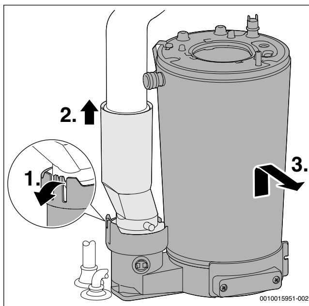
Fig. 65 Demontarea schimbatorului de căldură
