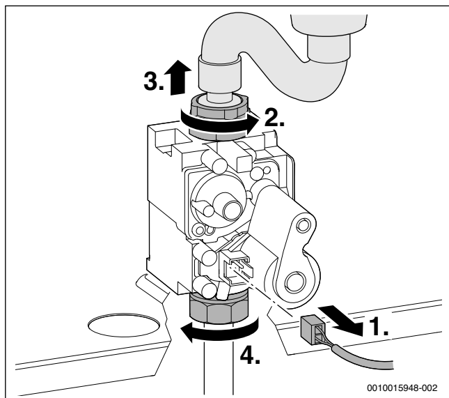
Fig. 59 Scoaterea șteccherului și desfacerea piulițelor oarbe
