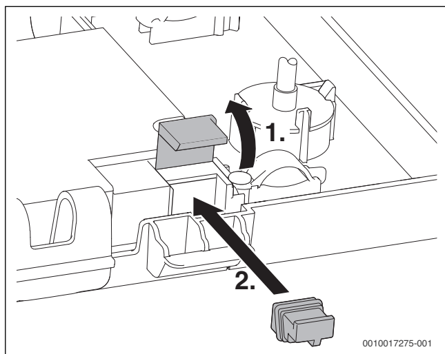
Fig. 67 Introduceți ștecărul de codare
