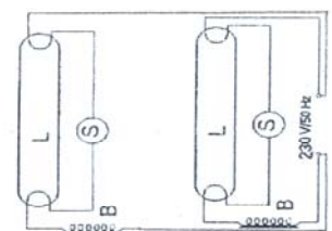
Fig. 2 Schema electrica
