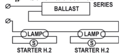
Fig. 2 Schema electrica
