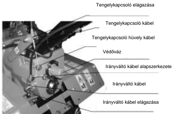
6. Ábra – Tengelykapcsoló kar felszerelése és beállítása
