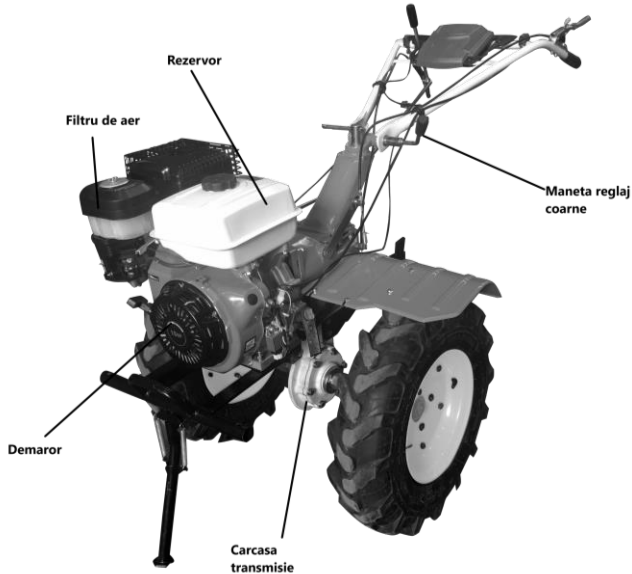
Fig. 4 – Montarea elementelor motosăpătoarei
