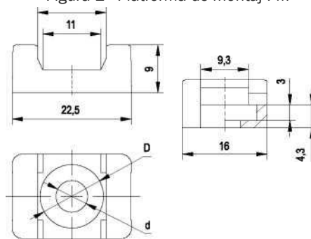
Figura 1 - Platformă de montaj PM
