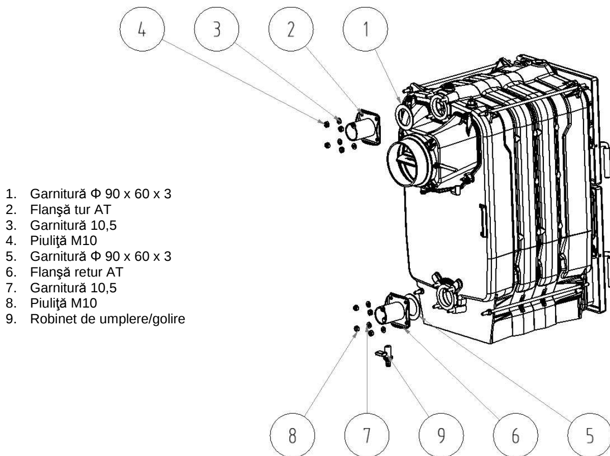
Fig. Nr. 15 Instalarea corpului de fontă a cazanului
