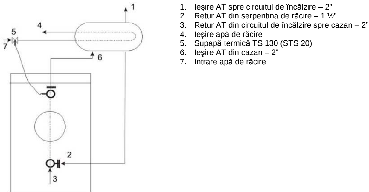
Fig. Nr. 6 Conexiunea hidraulică a serpentinei de răcire
