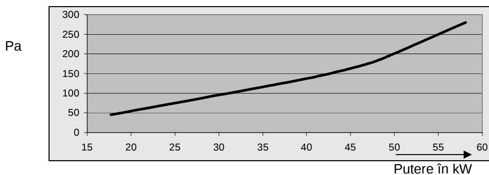
Fig. Nr. 1 Pierderile hidraulice în funcție de puterea cazanului
