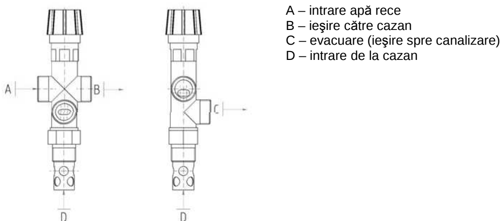
Fig. Nr. 7 Valva de siguranță cu 2 căi tip DBV 1 – 02
