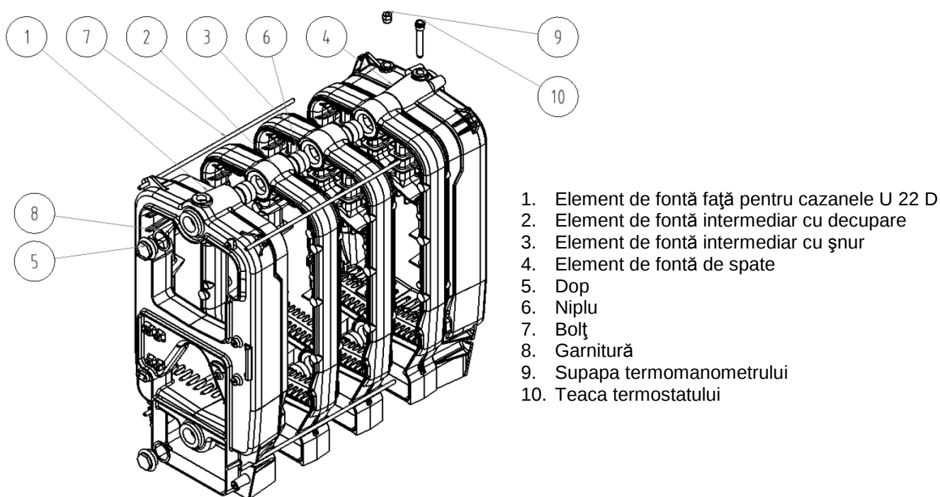
Fig. Nr. 3 Diagrama corpului de fontă pentru cazanele Viadrus Hercules U22D
