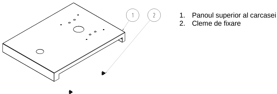
Fig. Nr. 22 Panoul superior al carcasei la cazanele prevăzute cu cutie de comandă
