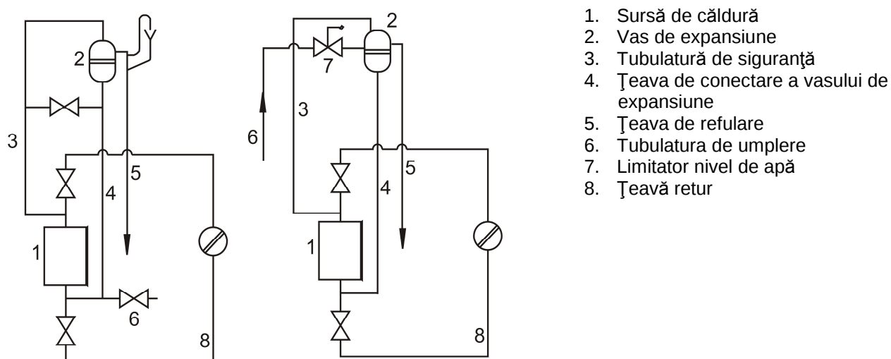
Fig. Nr. 9 Exemple de conectare a vasului de expansiune deschis
