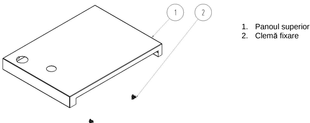
Fig. Nr. 19 Panoul superior a carcasei la cazanele fără cutie de comandă
