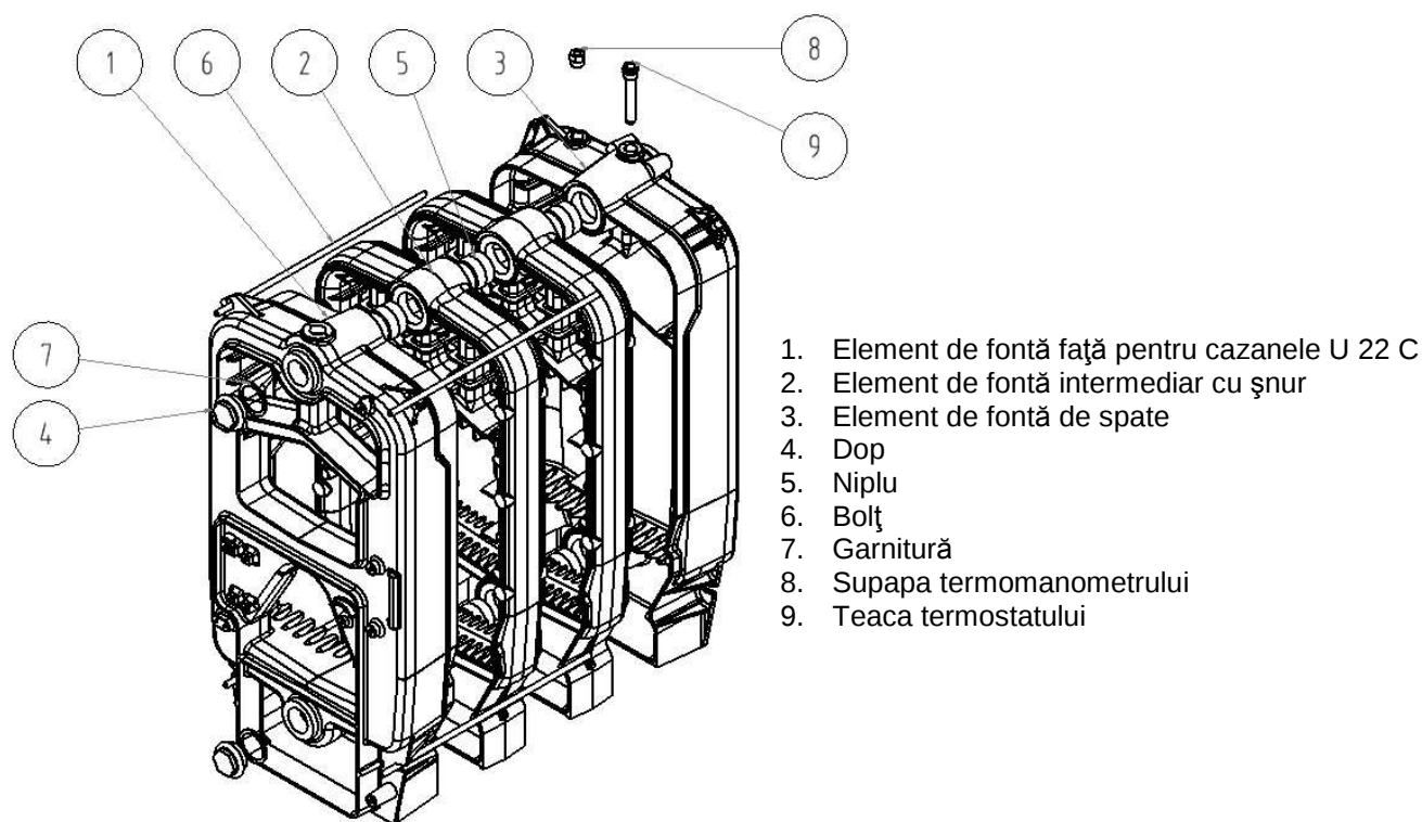
Fig. Nr. 2 Diagrama corpului de fontă pentru cazanele Viadrus Hercules U22C
