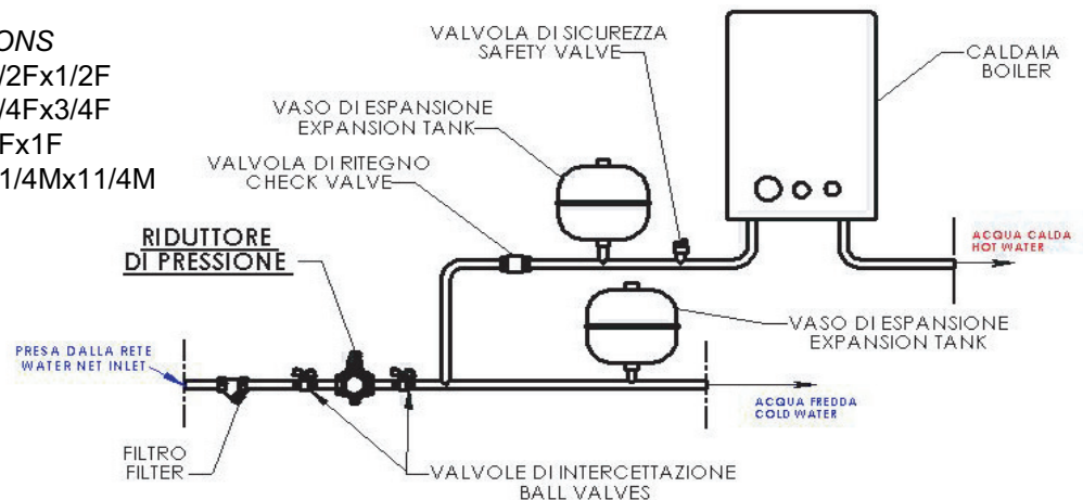
INSTALLAZIONE DI UN RIDUTTORE DI PRESSIONE CON CALDAIA
